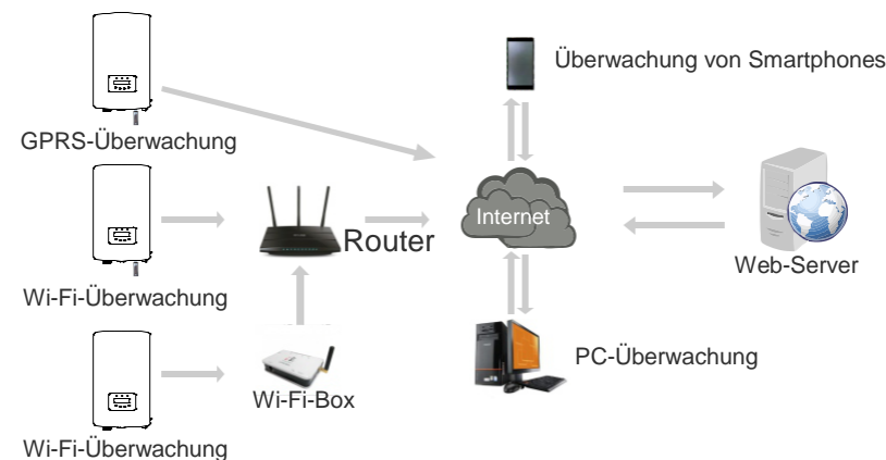
Abbildung 4.20 Wi-Fi- oder GPRS-Kommunikationsfunktion
