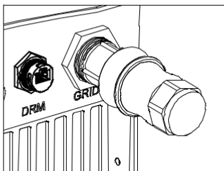
Abbildung 4.18 Anschluss des AC-Steckers an den Wechselrichter
