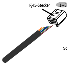
Abbildung 4.28 Abisolieren der Isolierschicht und Anschluss an RJ45-Stecker
